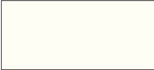
RAL 9010 Reinweiß
